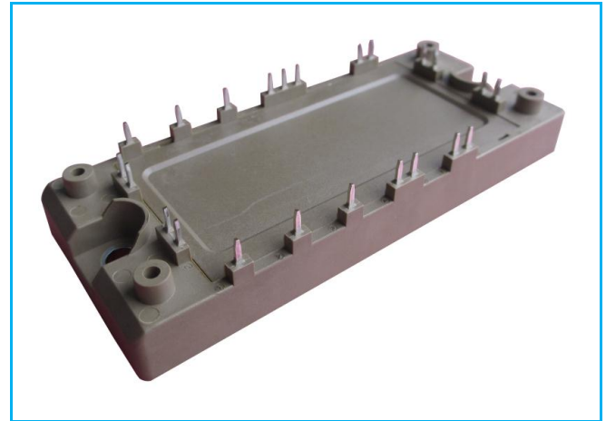
Rectifier+Brake+Inverter
